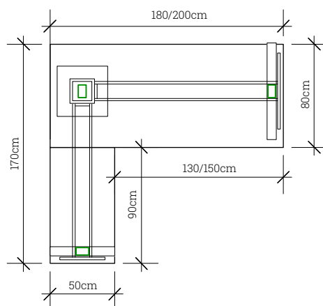
pianta - penisola a sx
